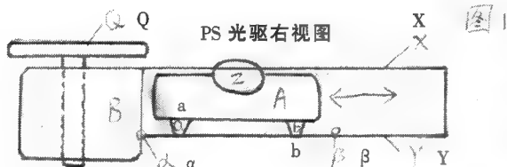
A: 光驱的整个光头部分。 Q: 光碟托盘。 Z: 悬空的光头物镜。 B: 光驱主马达。 a、b: 光头两滑动点。 x、y: 滑槽的顶线与底线。 \alpha 、 \beta : Y 线内侧能贴上胶布的两最外点。
